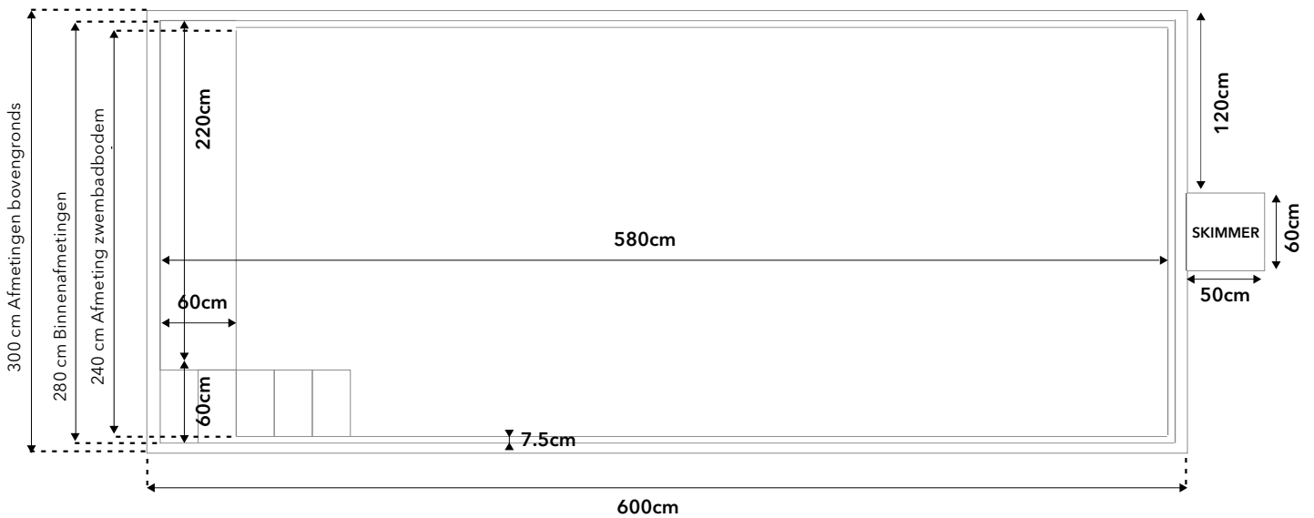
Zijaanzicht
